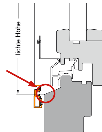
Unterkante des Blendrahmens bei Holzfenster flächenversetzt
