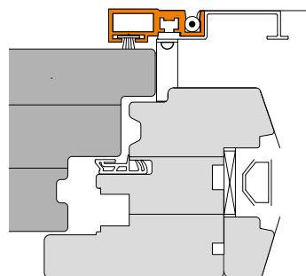
1) Stulpfensteranlage im Horizontalschnitt
