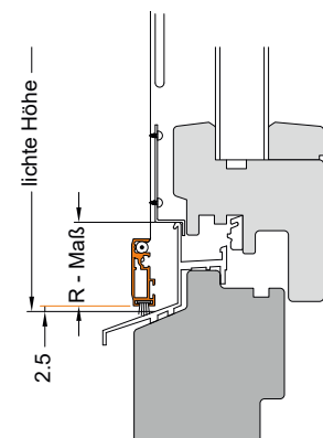
R-Maß bei Holzfenster mit Stockabdeckung
